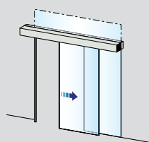
Montaža na letvu, vrata i bočne stijene (opcionalno gornje svjetlo)
