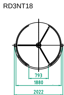
Top view, open door
