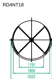
Top view, open door
